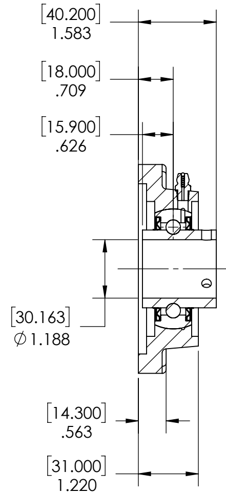
SECTION A-A
